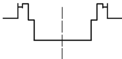
Z kątownikiem brzegowym pod dylatację od posadzki
